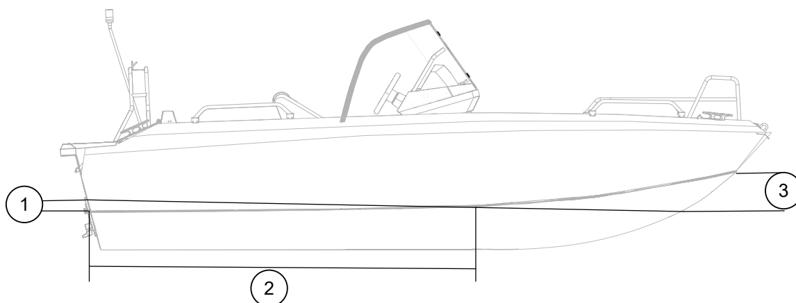
Figur 3.1 Bunnstoffområde for Buster LX
