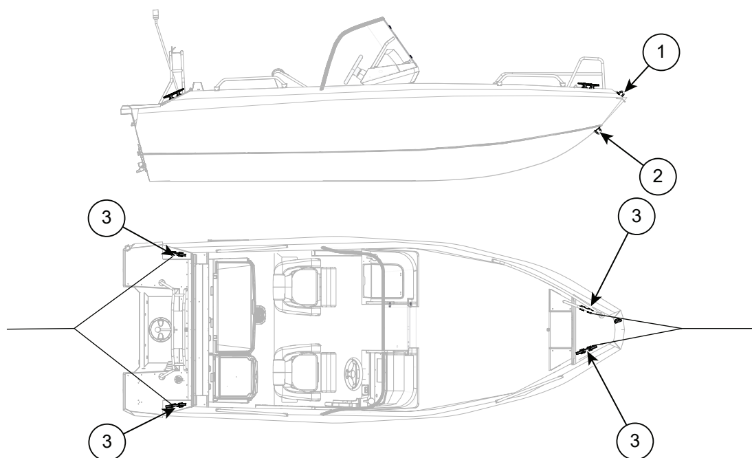
Figur 5.4 Fortøynings- og slepepunkter for Buster LX
