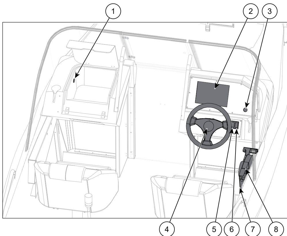
Figur 5.1 Styrestasjonskontroller for Buster LX
