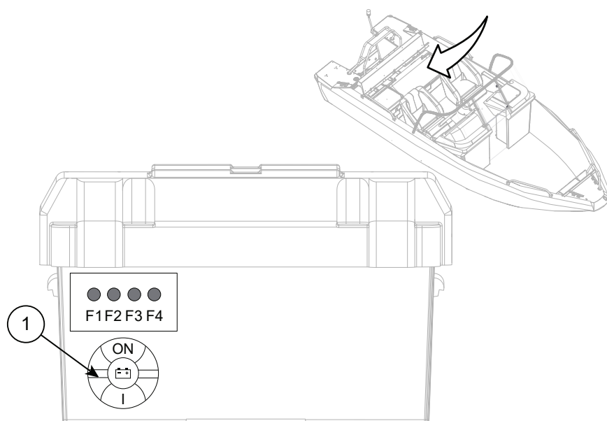
Figur 8.1 Hovedbryter og sikringspanel i Buster LX
